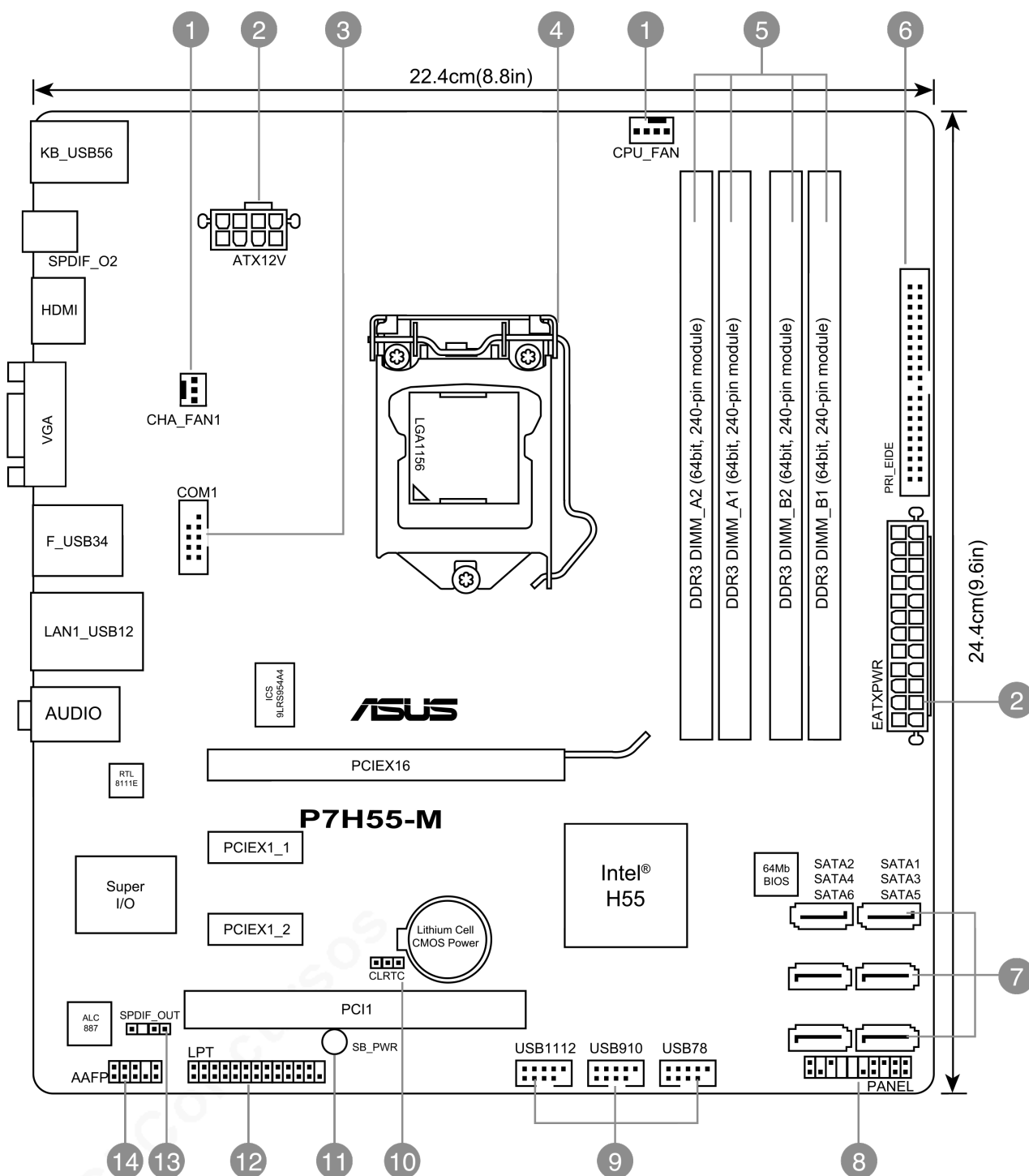
Figura: diagrama de componentes de placa mãe. Fonte: www.asus.com .
