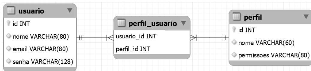
Figura: diagrama de entidades e relacionamentos entre usuários e seus perfis.
